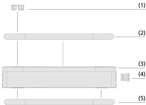
Systemaufbau Multi-Clamp Saugplatten VC-M-SP / VC-M-SPV
